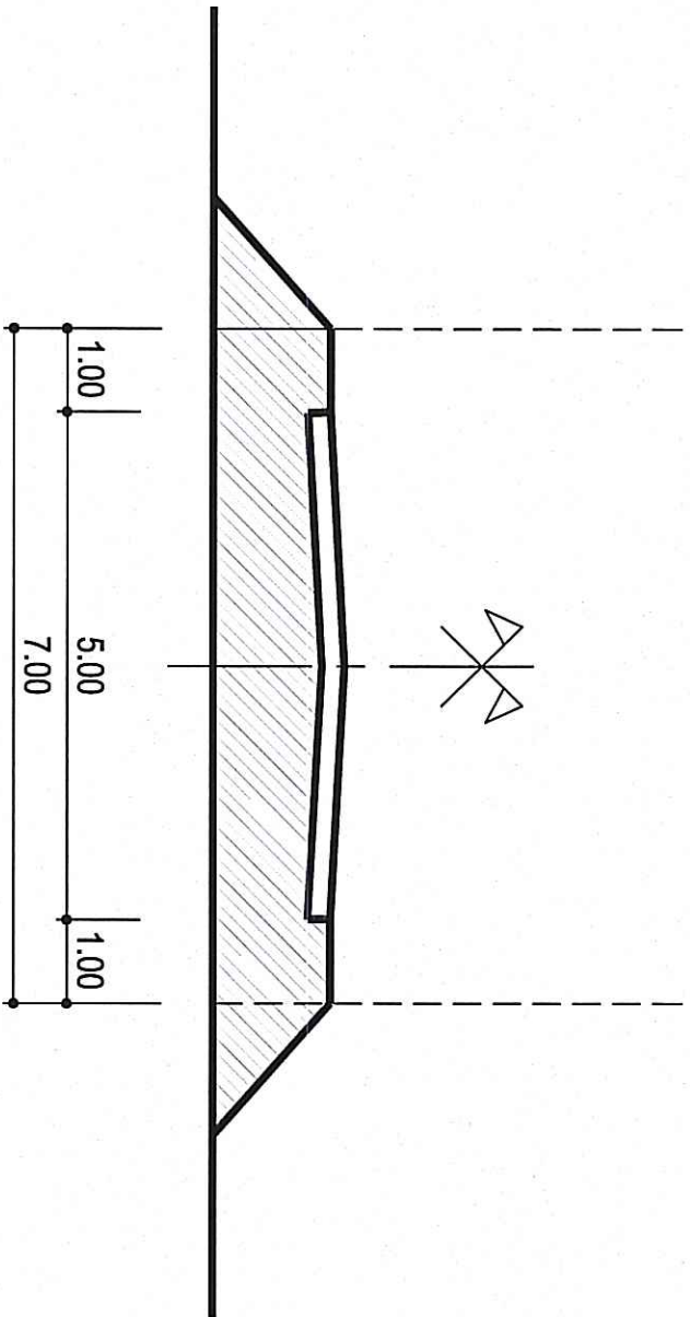
MẶT CẮT 2-2
